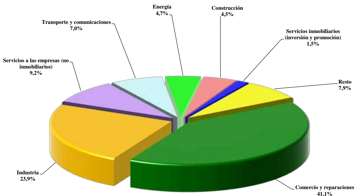
Gráfico 56 ESTRUCTURA DE LA SUMA DE DEDUCCIONES DEL REGIMEN GENERAL DEL IVA 2014, POR AGRUPACIONES DE SECTORES ECONÓMICOS
